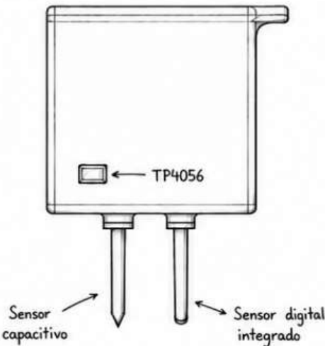
VISTA DE LA TAPA.
